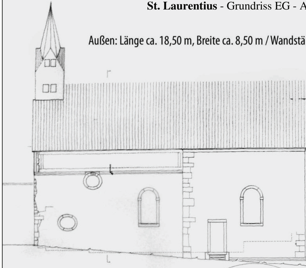
LÄNGSANSICHT SÜD
