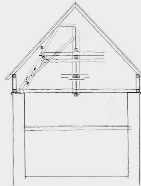
SCHNITT 1-1
