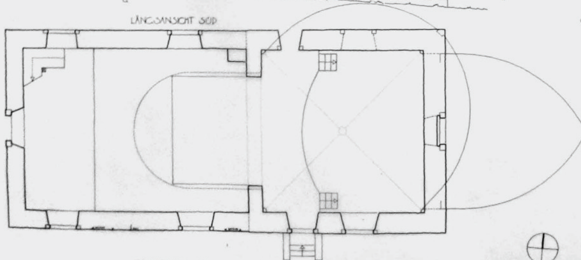
GRUNDRISS EG
